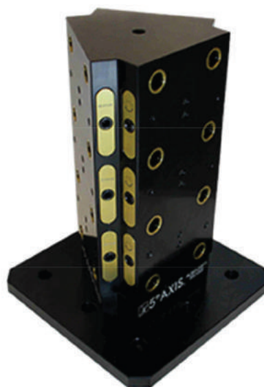
RL96A-3003 | RL96S-3003 Tour à trois faces pour 6X RL 96mm, sur base de 300 mm 2
